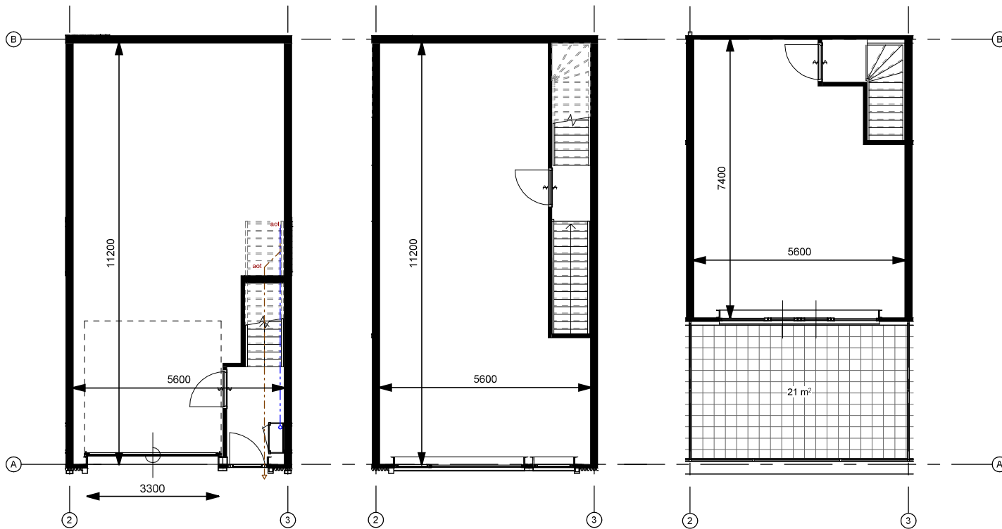
begane grond
