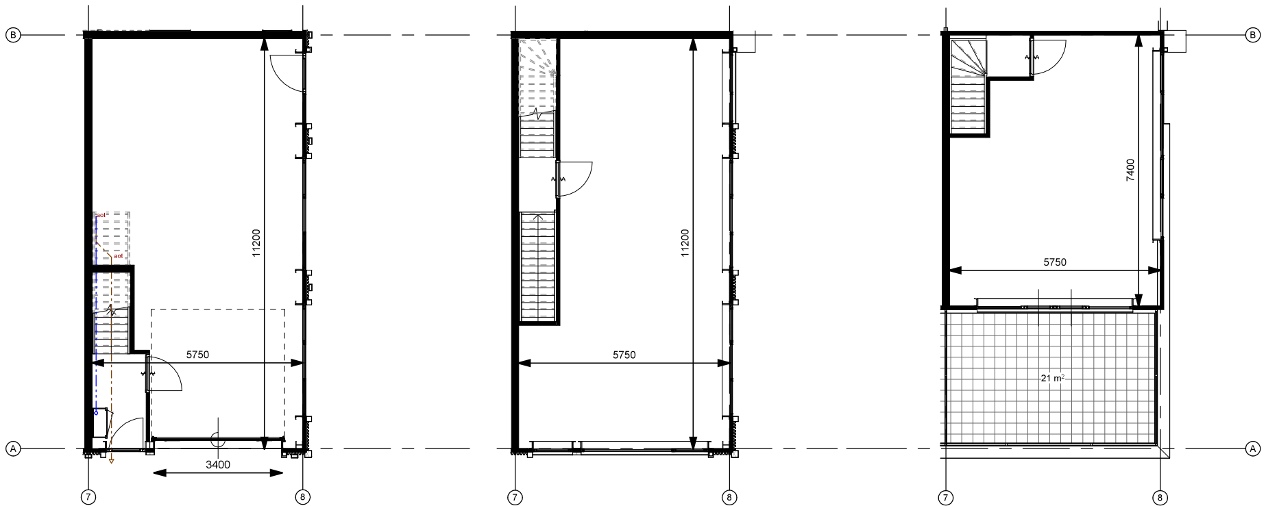
begane grond
