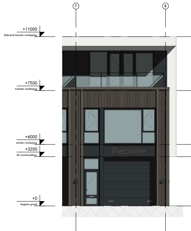
voorgevel
