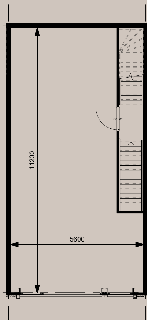
eerste verdieping
