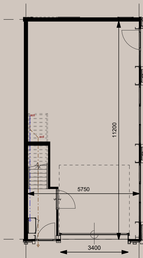
begane grond
