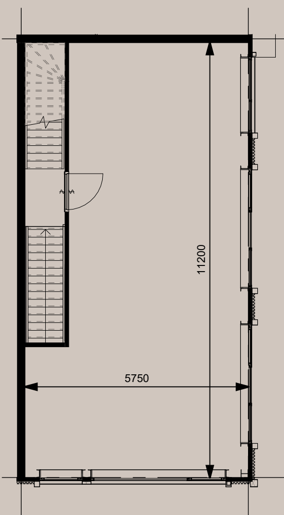
eerste verdieping
